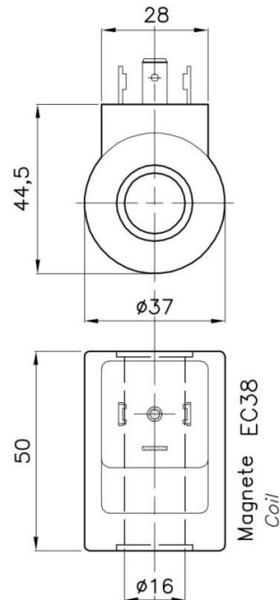
Габарити котушки С38
